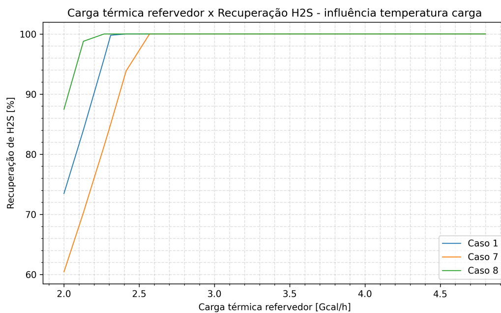
Figura 7: Carga térmica x recuperação de H 2 S - Influência da temperatura da carga
