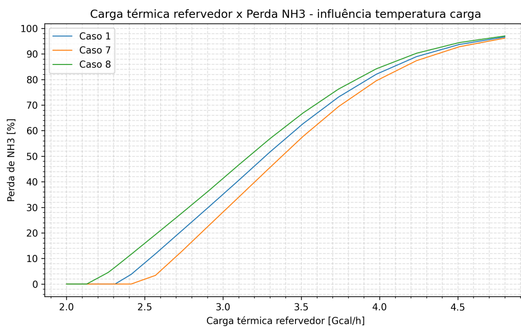
Figura 8: Carga térmica x perda de NH 3 - Influência da temperatura da carga
